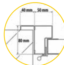
Dimensions du cadre
